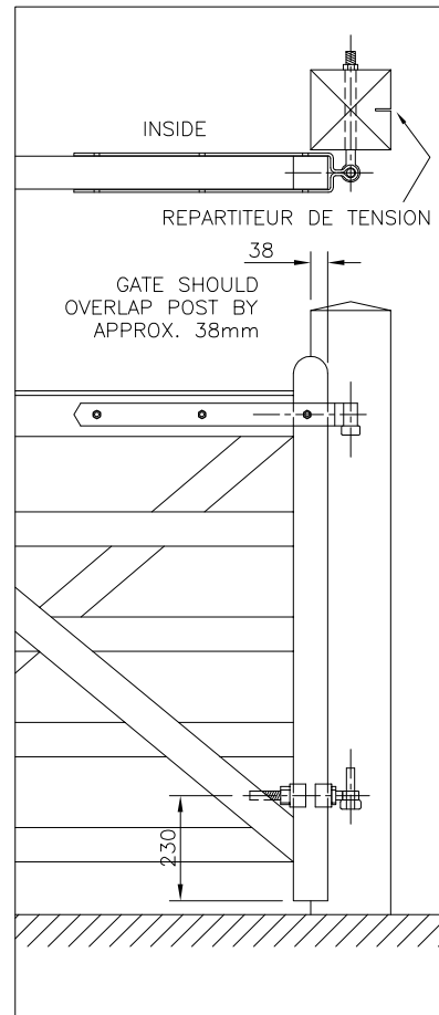
ACCROCHAGE A L'ARRIERE DES POTEAUX
