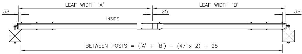
ACCROCHAGE A L'ARRIERE DES POTEAUX
