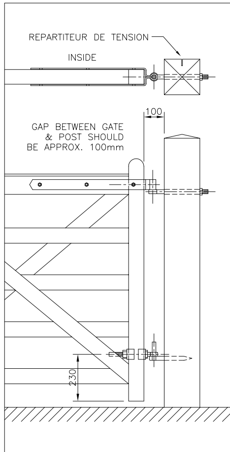
ACCROCHAGE ENTRE POTEAUX
