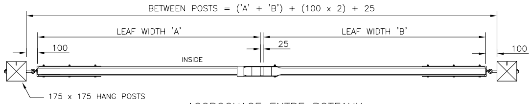
ACCROCHAGE ENTRE POTEAUX
